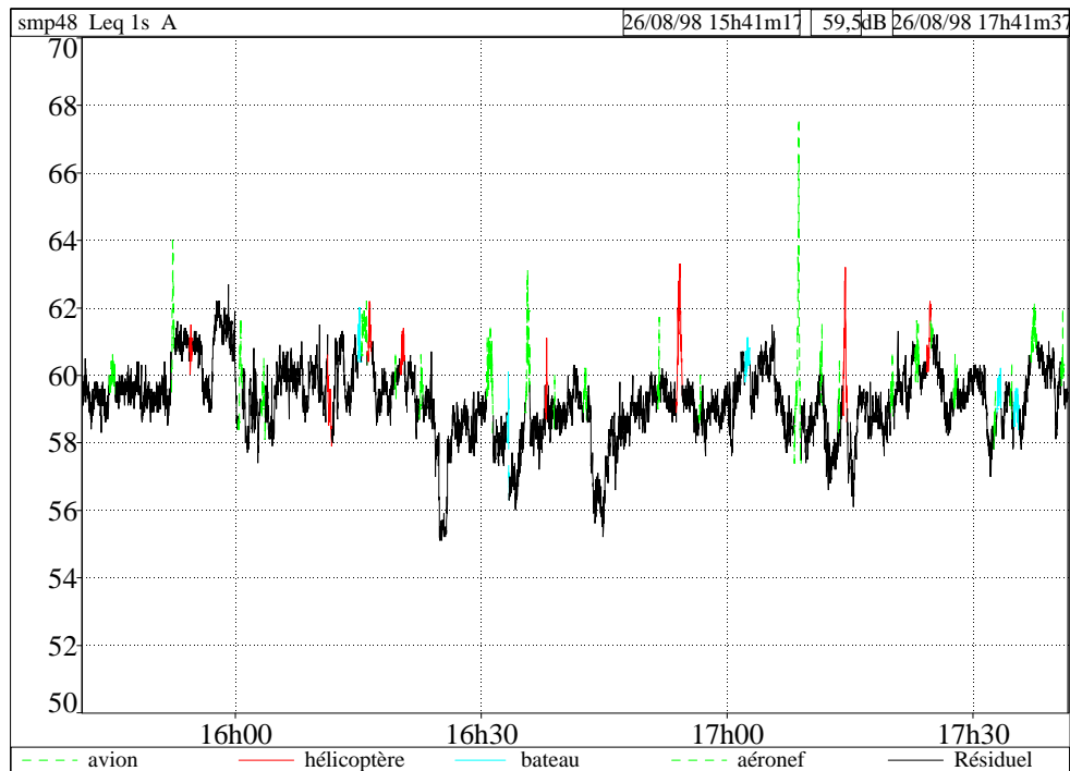
Représentation temporelle du signal acoustique et identification des sources sonores
