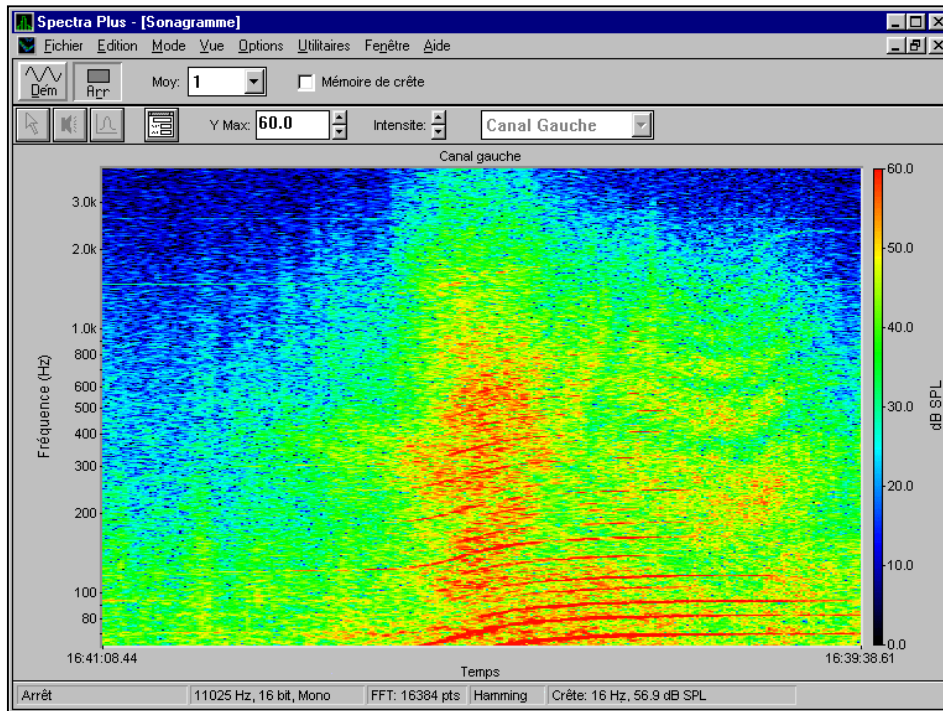
Signature acoustique du passage d'un hélicoptère
