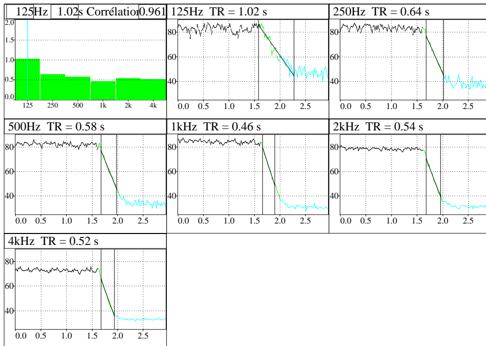
Exemple de calcul de la durée de réverbération par bandes d'octave
