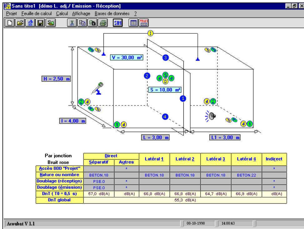
Exemple de calcul d'isolement acoustique entre deux logements
