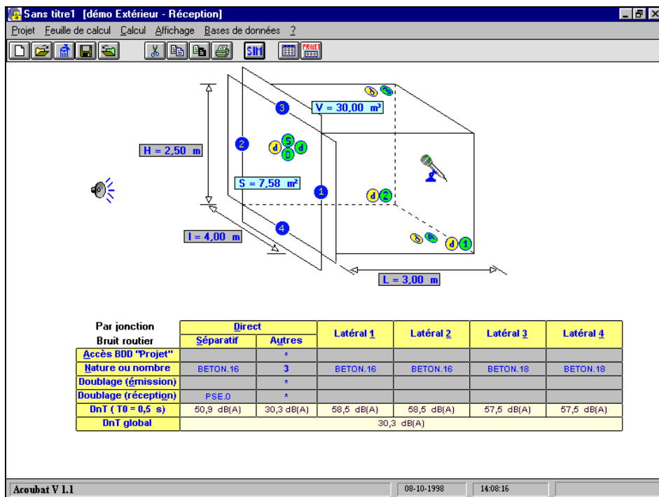
Exemple de calcul d'isolement de façade
