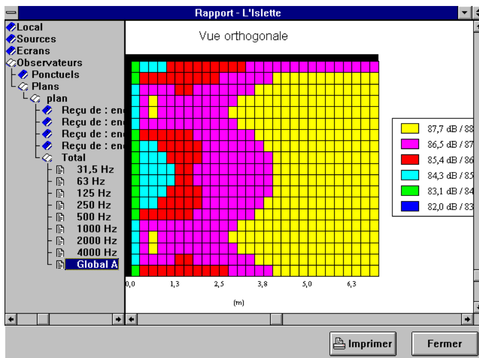
Exemple de cartographie des niveaux sonores à l'intérieur d'un local
